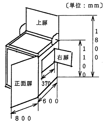
専用ボックス主要寸法
