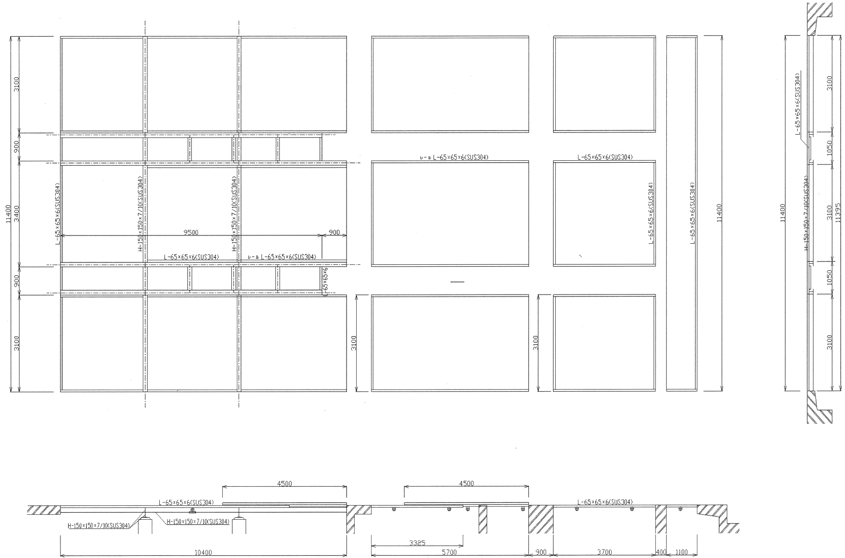
No.8 最初沈殿池受枠詳細図
