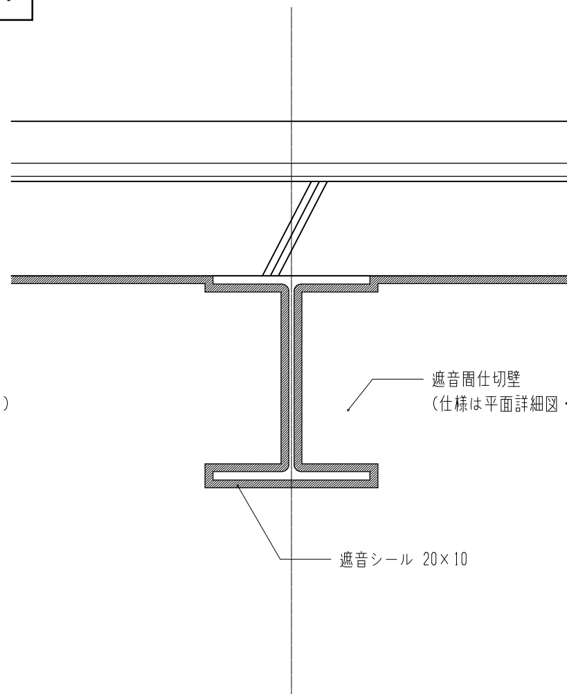
遮音間仕切り梁貫通部詳細図 S=1/10(A4)
