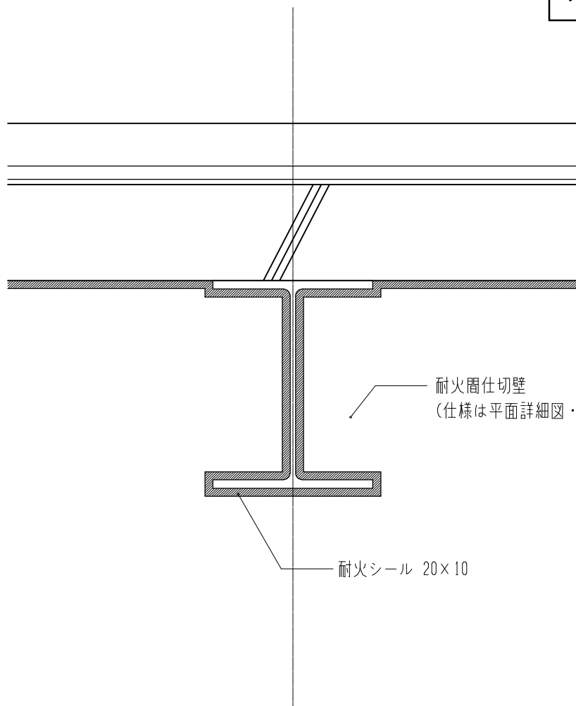
耐火間仕切り梁貫通部詳細図 S=1/10(A4)
