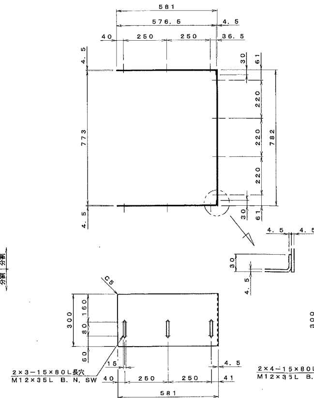
ウェアプレート詳細図 S=1/10
