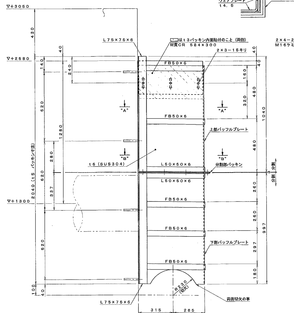
終沈バツフルプレート詳細図 S=1/10
