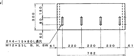
ウェアプレート詳細図 S=1/10
