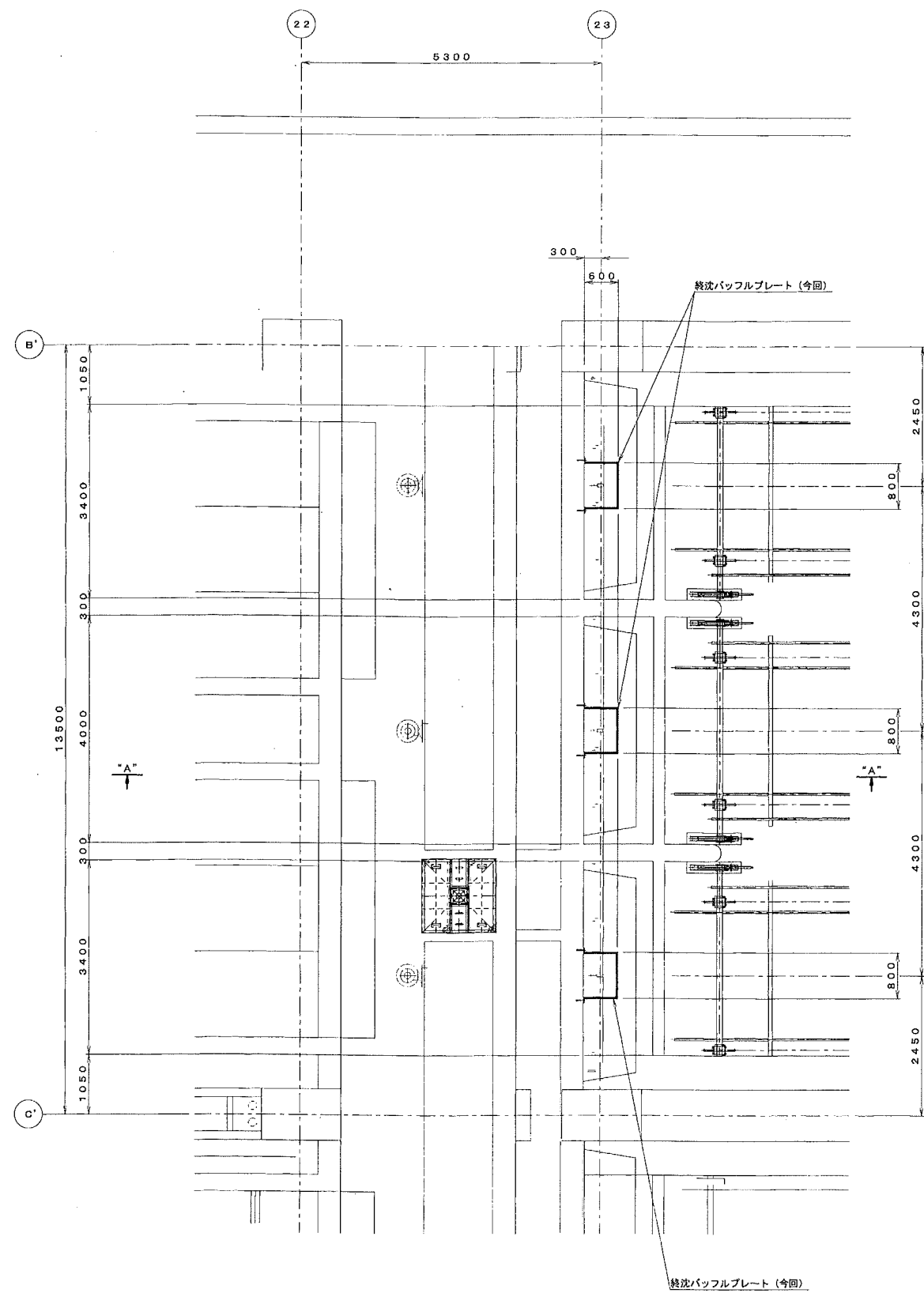
最終沈殿池上部平面図 S=1/50
