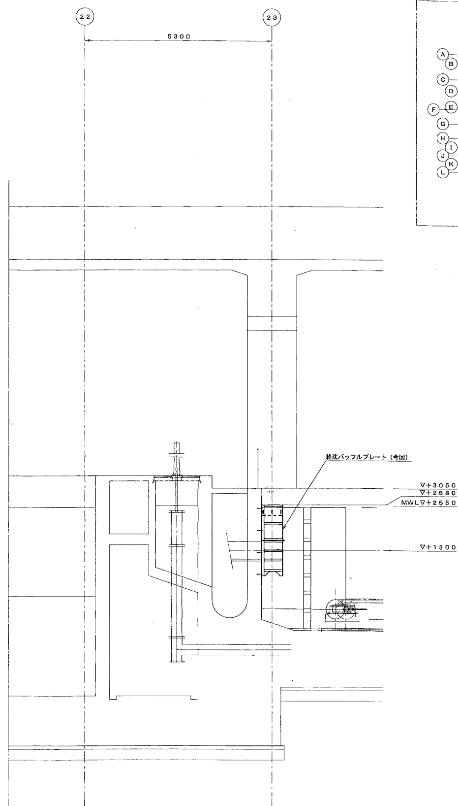
"A" - "A" 断面図 S=1/50
