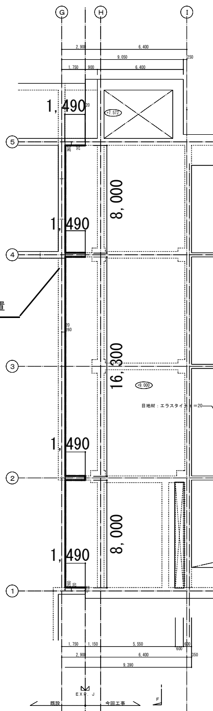
平面（下面）
