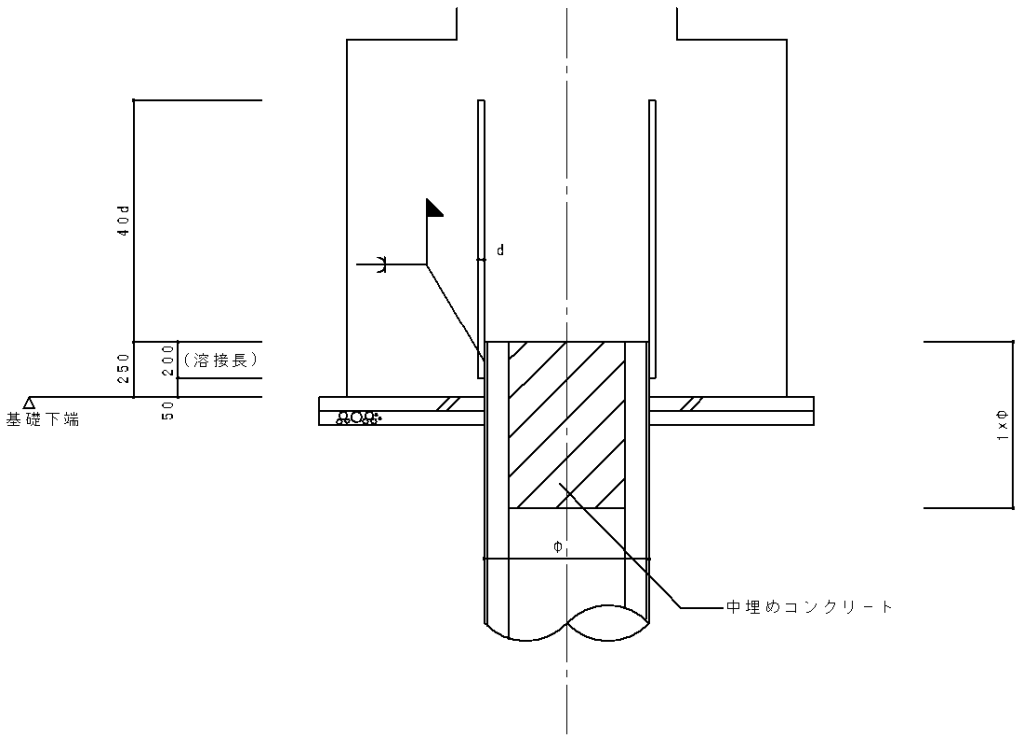
S C 杭頭補強筋要領図
